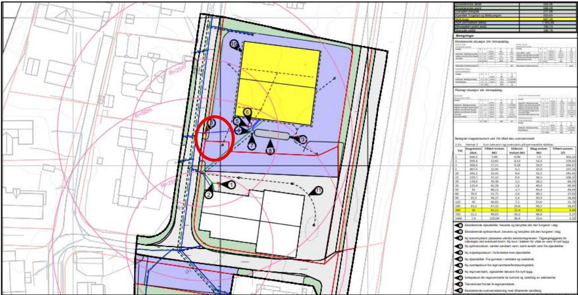
Figur12, Utlipp av VAO-plan, med plassering av ny hydrant. Plassering er innenfor 50 meters radius for både nytt og eksisterende bygg.
